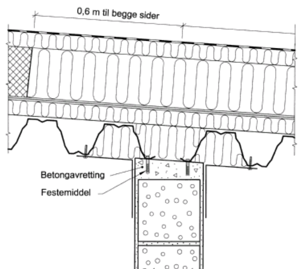
Fig. 27 Branncellebegrensende vegg avsluttet under bærende profilerte stålplater
