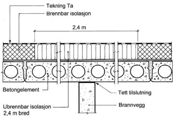
Fig. 29 Dekke av betongelement over seksjoneringsvegg eller brannvegg
