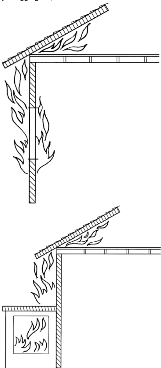
Fig. 39 Brannspredning fra underliggende rom til tak
