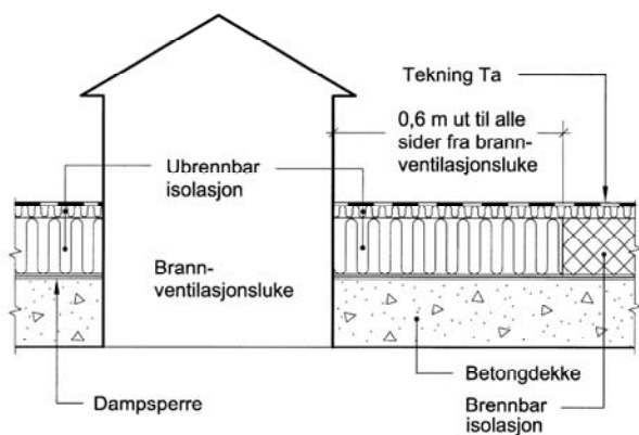
Fig. 18 Brannventilasjonslukke på betongdekke
