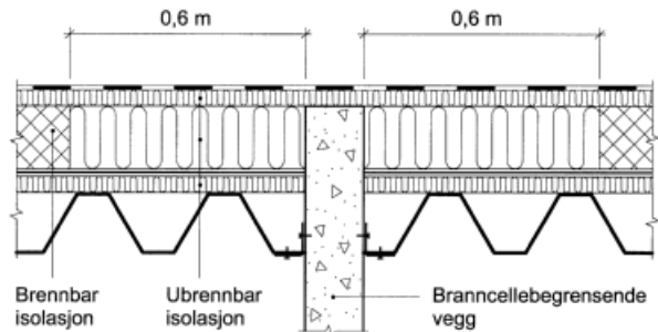
Fig. 26 Stålplatetak inntil branncellebegrensende vegg
