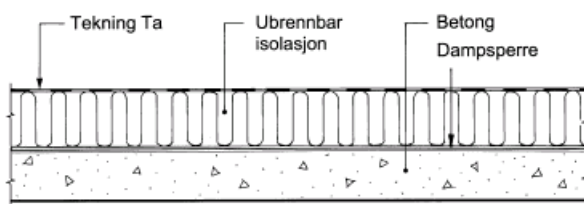
Fig. 5 Ubrennbar isolasjon på betongdekke
