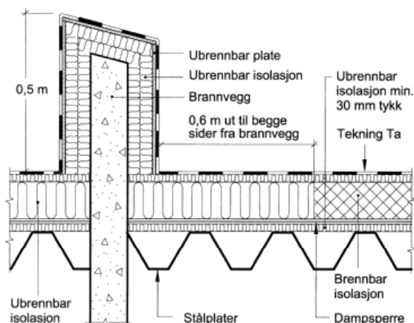
Fig. 33 Stålplatetak inntil seksjoneringsvegg eller brannvegg
