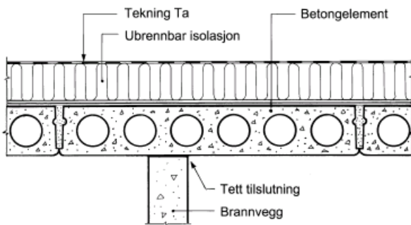
Fig. 28 Dekke av betongelement over seksjoneringsvegg eller brannvegg
