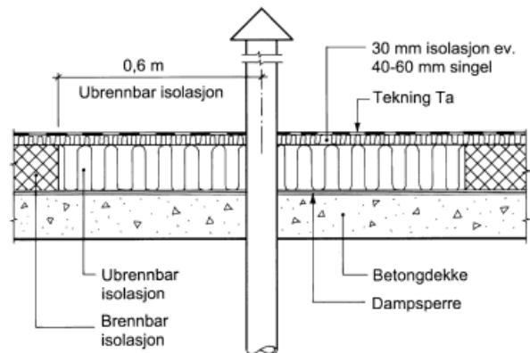
Fig. 19 Gjennomføring i betongdekke med brennbar isolasjon
