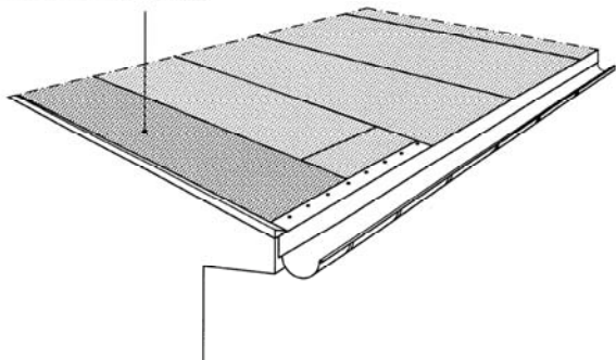
Fig. 45 Gavl på ventilerte takflater Tildekkes med underlagsbelegg i en bredde på minimum 1 m før bruk av åpen flamme. I stedet kan sveising med varmluft benyttes.
