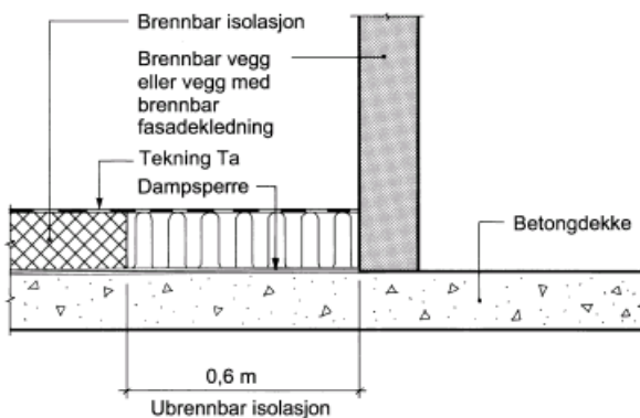
Fig. 25 Tak mot brennbar vegg
