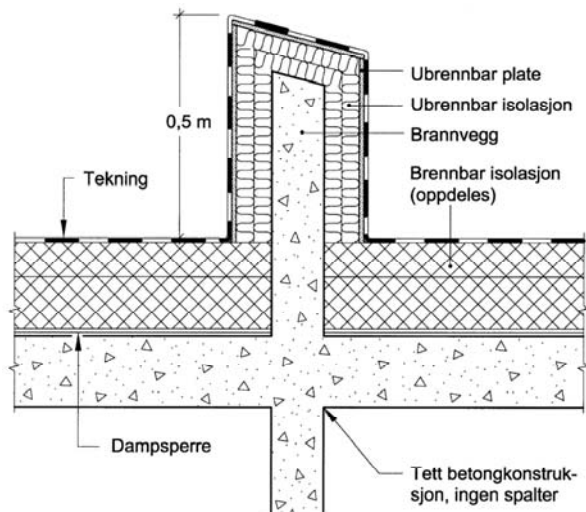
Fig. 34 Plasstøpt betongkonstruksjon med seksjoneringsvegg eller brannvegg
