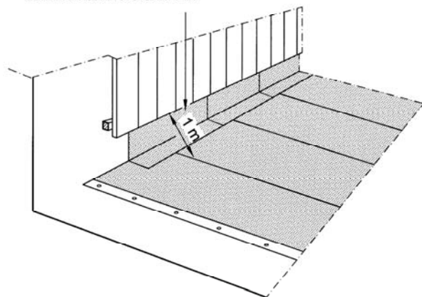
Fig. 41 Under utlektet kledning på vegg
