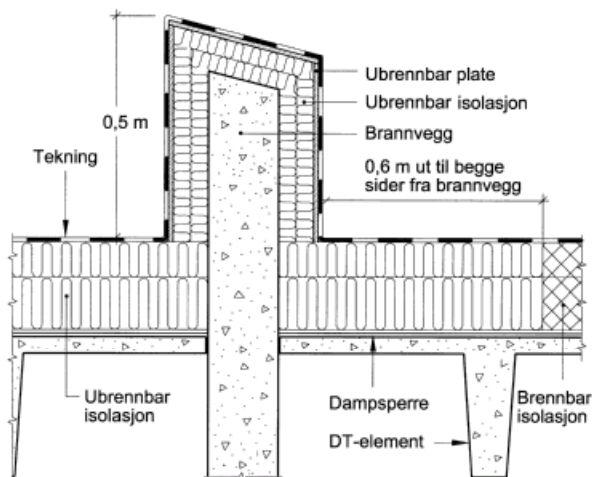
Fig. 32 DT-element inntil seksjoneringsvegg eller brannvegg
