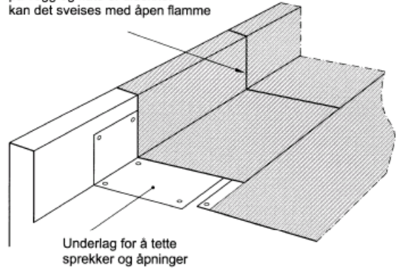
Fig. 42 Andre oppkanter
