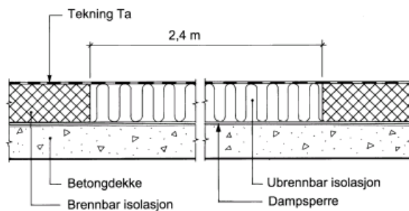
Fig. 7 Brennbar isolasjon på betongdekke med oppdeling
