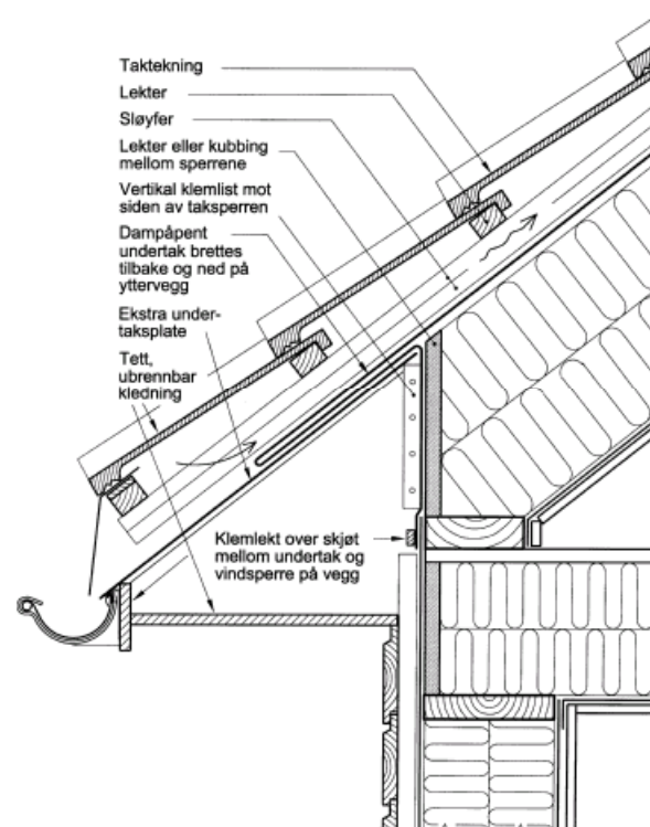
Fig. 40 Isolert skråtak bør velges istedenfor kaldt loft
