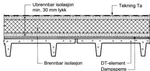
Fig. 9 Brennbar isolasjon på DT-elementer
