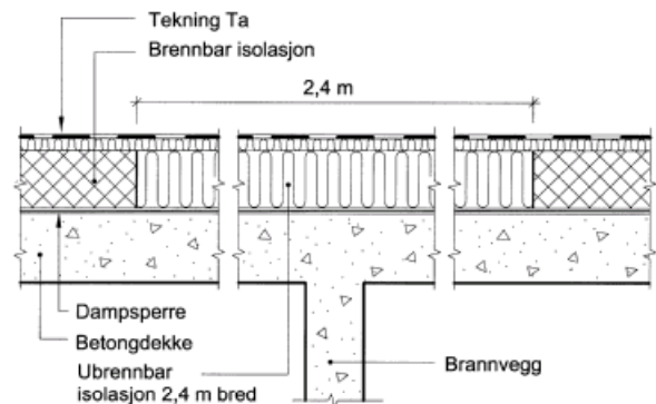
Fig. 31 Betongdekke over brannvegg eller seksjoneringsvegg
