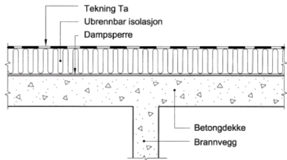
Fig. 30 Betongdekke over seksjoneringsvegg eller brannvegg
