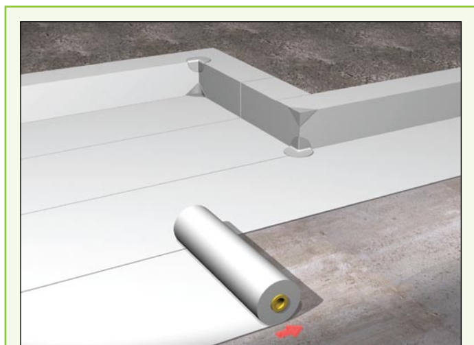
Protan RadonSafe kan monteres både i bruksgruppe B og C. Omleggene sammenføres ved varmluftsveisede skjøter. Dette sikrer god radontetthet.
