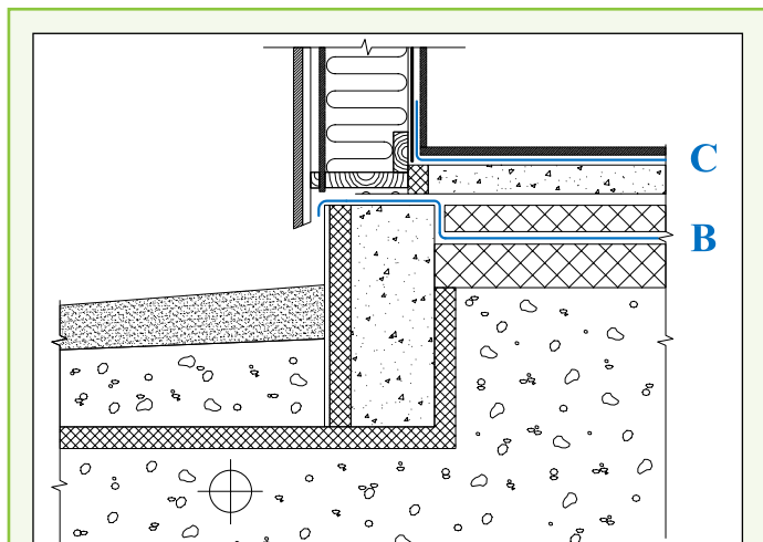
Prinsippkisse for plassering av Protan RadonSafe i bruksklasse B og C.
